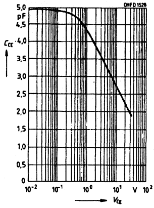
Capacitance C_{CE}=f(V) , f=1\text{ MHz} , E=0
