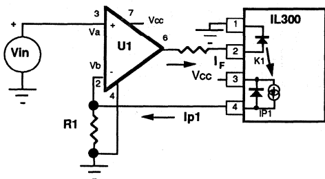
Figure 5. Optial Servo Amplifiert
