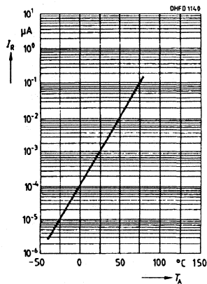
Dark current I_R=f(T_A) , E=0 , V_R=20V
