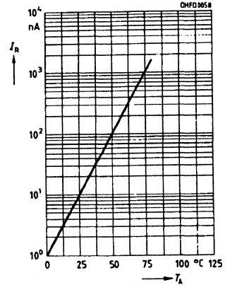
Dark current I_R=f(T_A) , V_R=10 V
