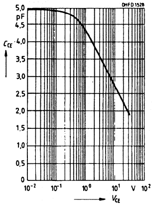
Capacitance C_{CE}=f(V_{CE}) , f=1 MHz, E=0
