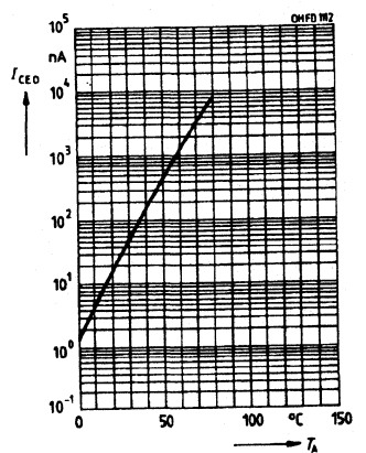
Dark current-BPX81 I_{CEO}=f(T_A) , V_{CE}=25\text{ V} , E=0
