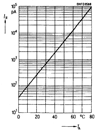
Dark current I_R=f(T_A) , V_R=7\text{ V} , E=0
