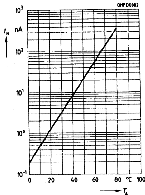
Dark current I_R=f(T_A) V_R=10, E=0
