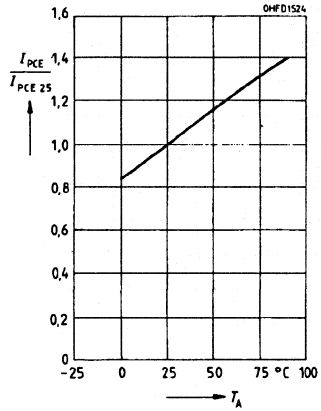
Dark current I_{PCE}/I_{PCE25}=f(T_A) , V_{CE}=25 V
