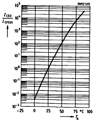
Dark current I_{CE0}/I_{CE025}=f(T_A) , V_{CE}=25\text{ V} , E=0
