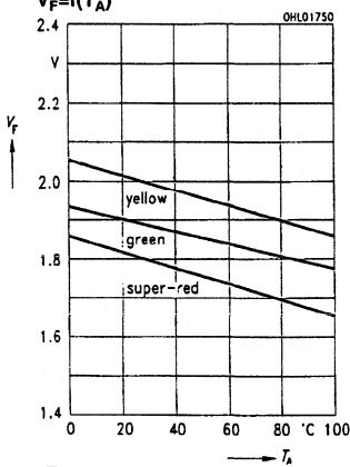
9E Forward voltage V_F=f(T_A)
