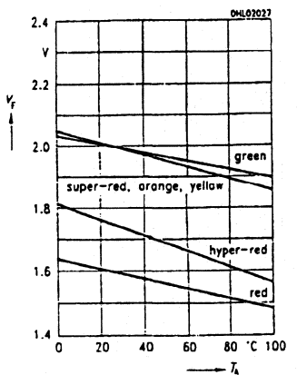
9A Forward voltage V_F=f(T_A)
