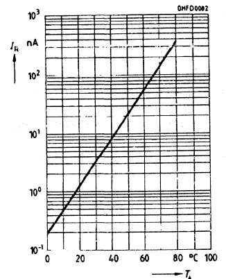
Dark current I_R=f(T_A) V_R=10, E=0
