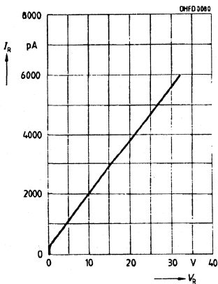
Dark current I_R=f(V_R) T_A=25^\circ C, E=0
