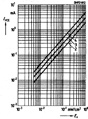
Photocurrent I_{PCE}=f(E_V) , V_{CE}=5\text{ V}
